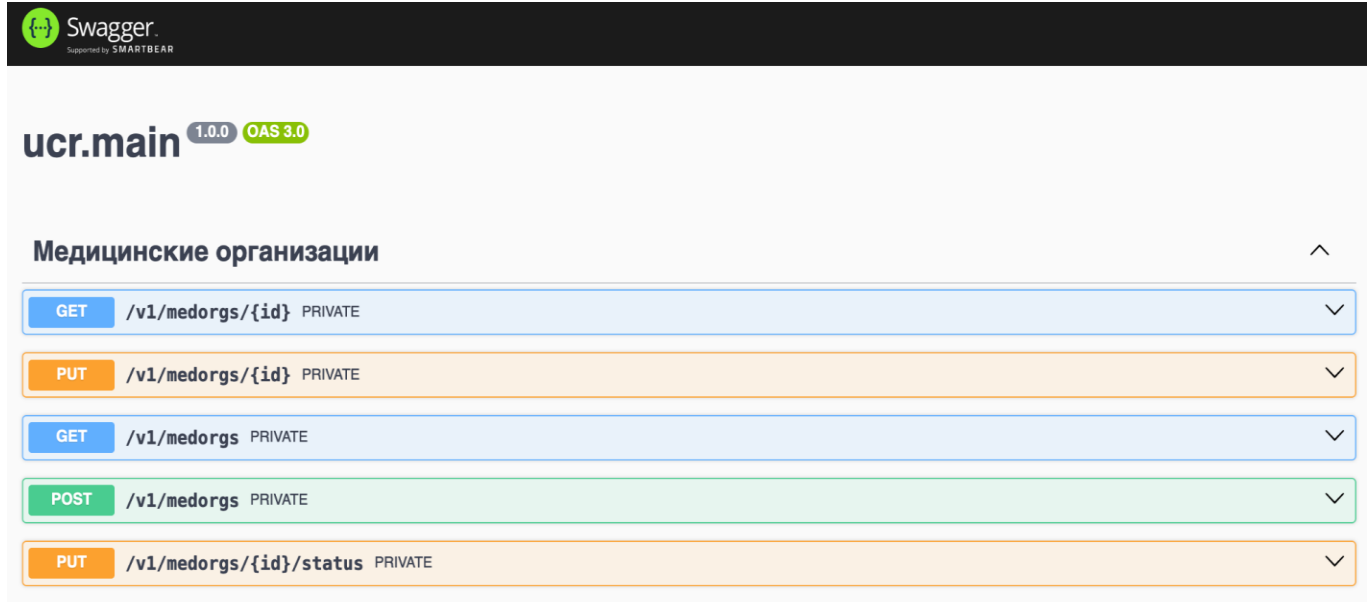
Рисунок 1 – Страница с описанием API в формате OpenAPI
